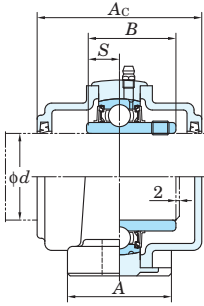
Con tapa de fundición gris
