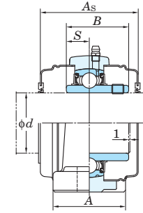
Con tapa de chapa de acero
