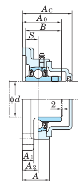
Con tapa de fundición gris
