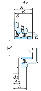
Con tapa de fundición gris
