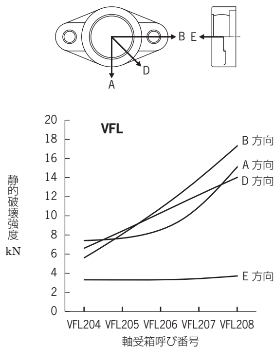
図 8.16 プラスチック製軸受箱(VFL)の静的破壊強度
