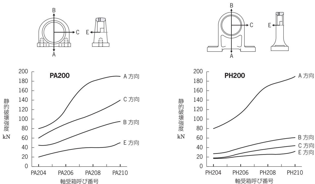
図 8.3 狭幅ピロー形軸受箱(PA)の静的破壊強度
