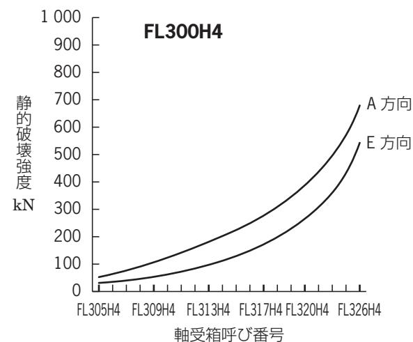
図 8.10 球状黒鉛鋳鉄製ひしフランジ形軸受箱(FLH4)の静的破壊強度
