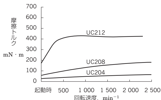
図 13.1 軸受ユニットの摩擦トルク測定結果例
