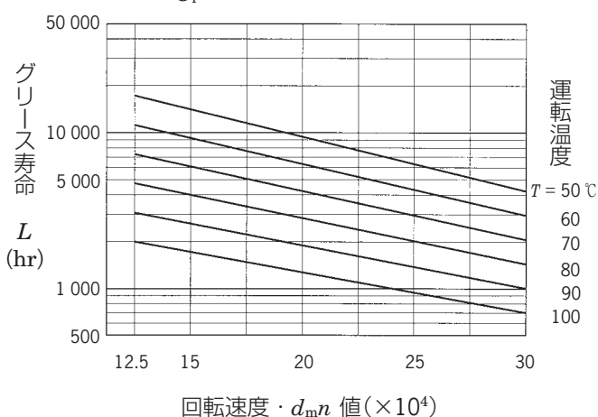
図 4.2 軸受荷重、回転速度および運転温度とグリース寿命の関係(参考)
