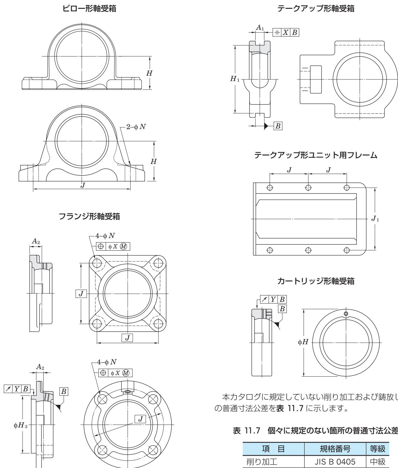
図 11.1 許容差および許容値を持つ軸受箱の取り付けに関する寸法(代表例)
