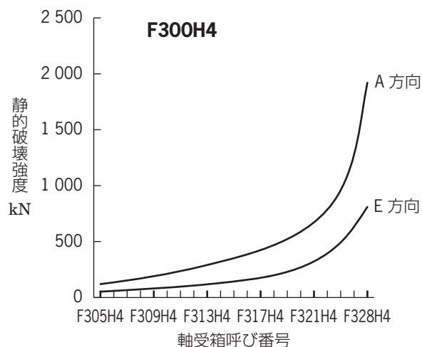
図 8.9 球状黒鉛鋳鉄製角フランジ形軸受箱(FH4)の静的破壊強度
